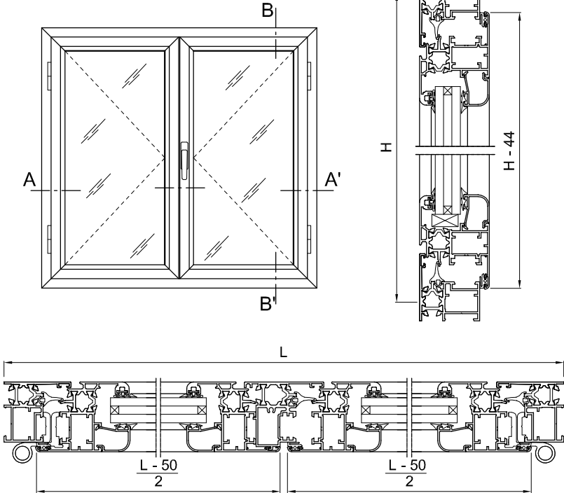
Sección A-A'
